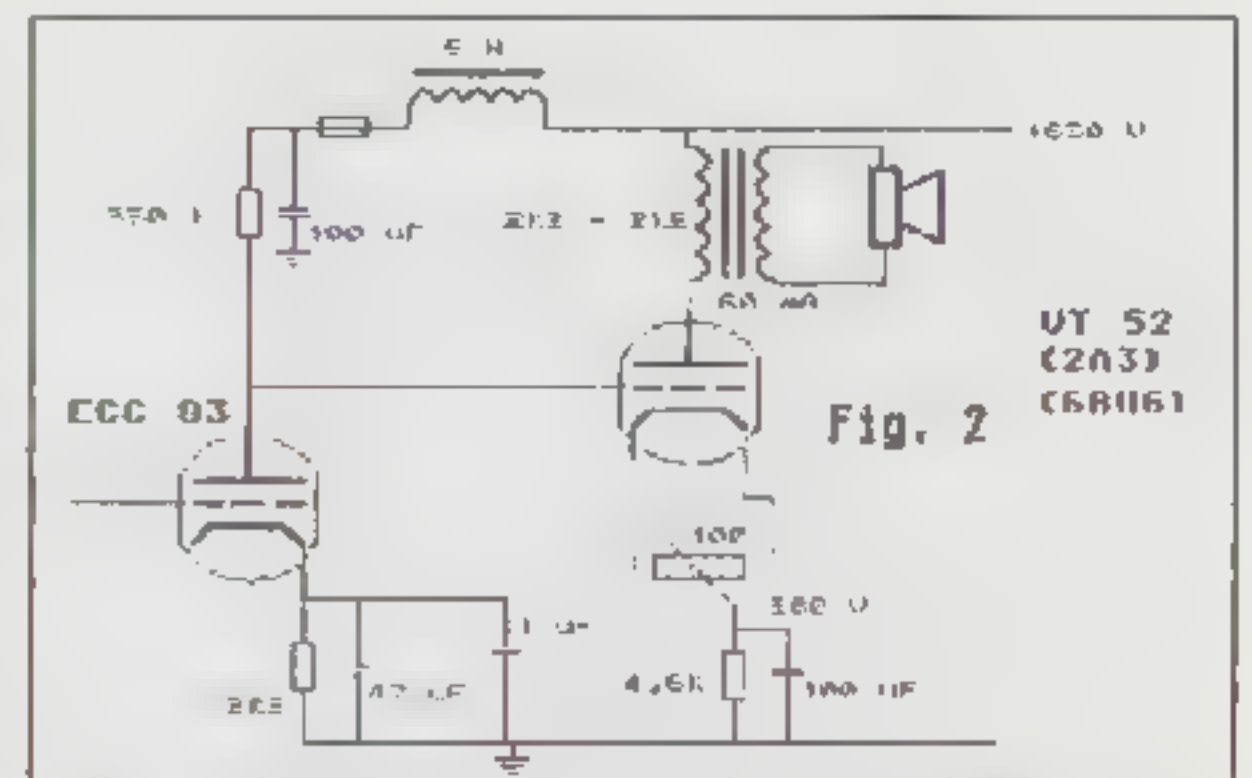
De schakeling van l'Audiophile uit 1977
